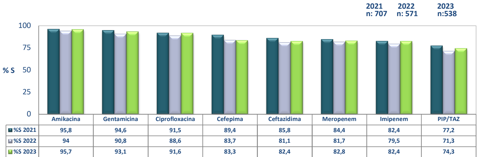
Perfiles de sensibilidad a antibióticos de Pseudomonas aeruginosa en UCI 2021-2023.
